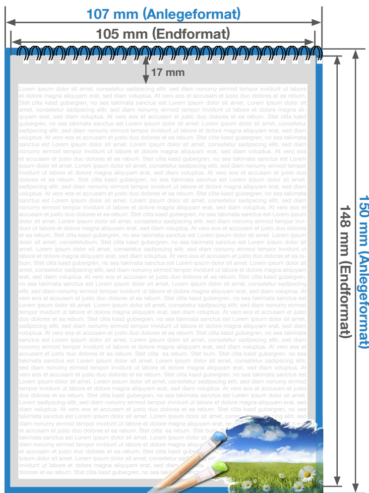
Zeichnung nicht maßstabgetreu
