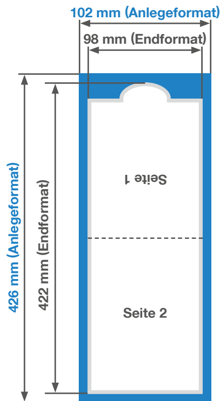
Zeichnung nicht maßstabsgetreu
